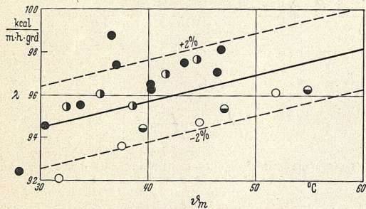
Abb. 8. Messing I (unbekannt) verglichen mit Stahl St 42.11 ○, Reinickel ○, Messing II ●, Aluminium ○
