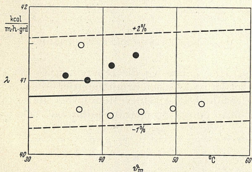
Abb. 6. Stahl St 42.11 I (unbekannt) verglichen mit Remanit ○ und Stahl St 42.11 II ●
