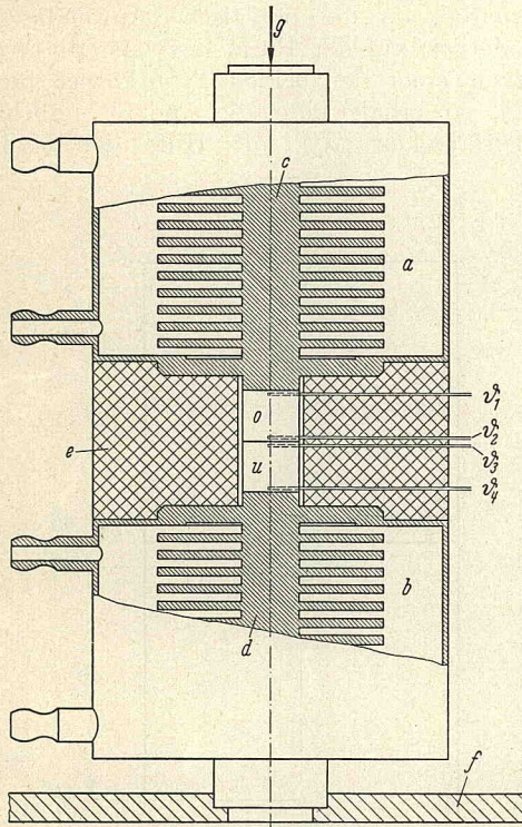
Abb. 2. Versuchseinrichtung. a Heizkammer, b Kühlkammer, c , d Messingstempel, e Wärmeschutzhülle aus Schaumstoff, f Stahlplatte, g Druckvorrichtung, o oberer Probekörper, u unterer Probekörper
