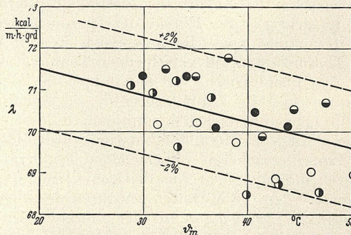
Abb. 7. Reinickel I (unbekannt) verglichen mit Stahl St 42.11 ○, Reinickel ●, Messing ○ und Aluminium ○
