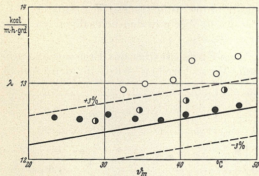
Abb. 5—9. Ermittlung der Wärmeleitfähigkeit verschiedener Metallproben mit Hilfe von Standardproben bekannter Wärmeleitfähigkeit
