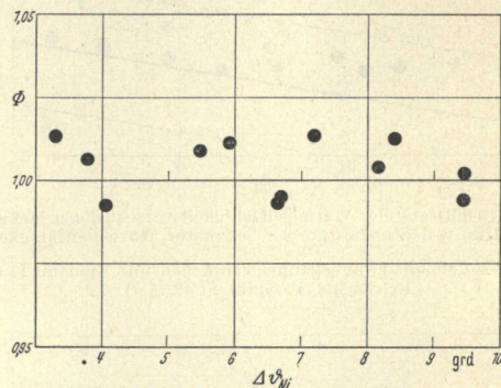
Abb. 3. Vergleich zweier Nickelproben I und II
