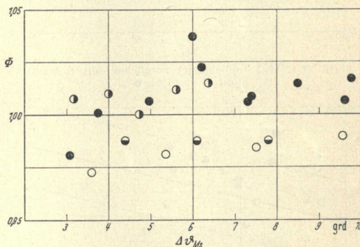
Abb. 4. Vergleich einer Messingprobe I mit Standardproben von Nickel \circ , Aluminium \bullet , Messing II \bullet und Stahl St 42.11 \ominus
