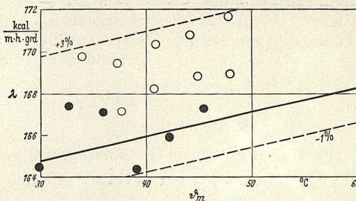
Abb. 9. Aluminium I (unbekannt) wird verglichen mit Messing ○ und Aluminium I ●
